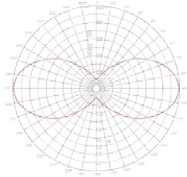
Peanut
